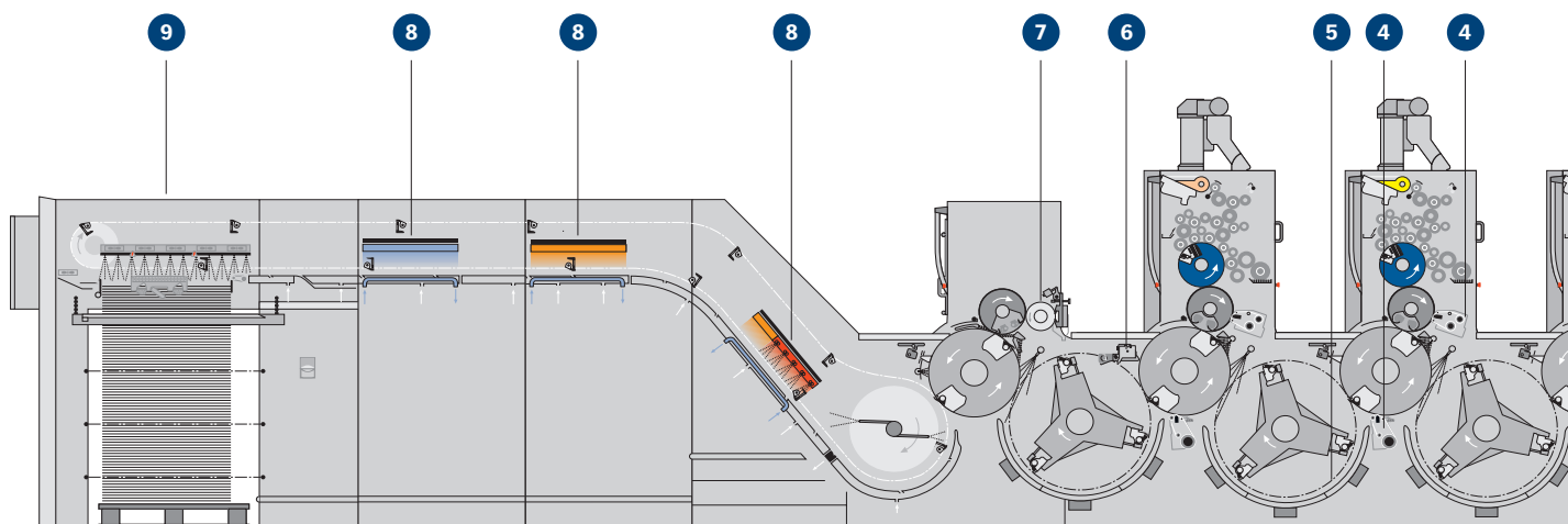
スピードマスター CX102-5+L の構成例 (オプション装置を含む)
