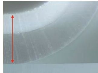
TPU 断面
